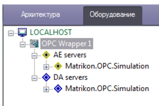
Рис. 3-2 Поиск OPC-серверов
