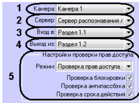
Рис. 2.2—3 Настройка точки прохода
