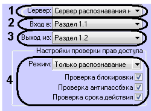
Рис. 2.1—3 Настройка точки прохода
