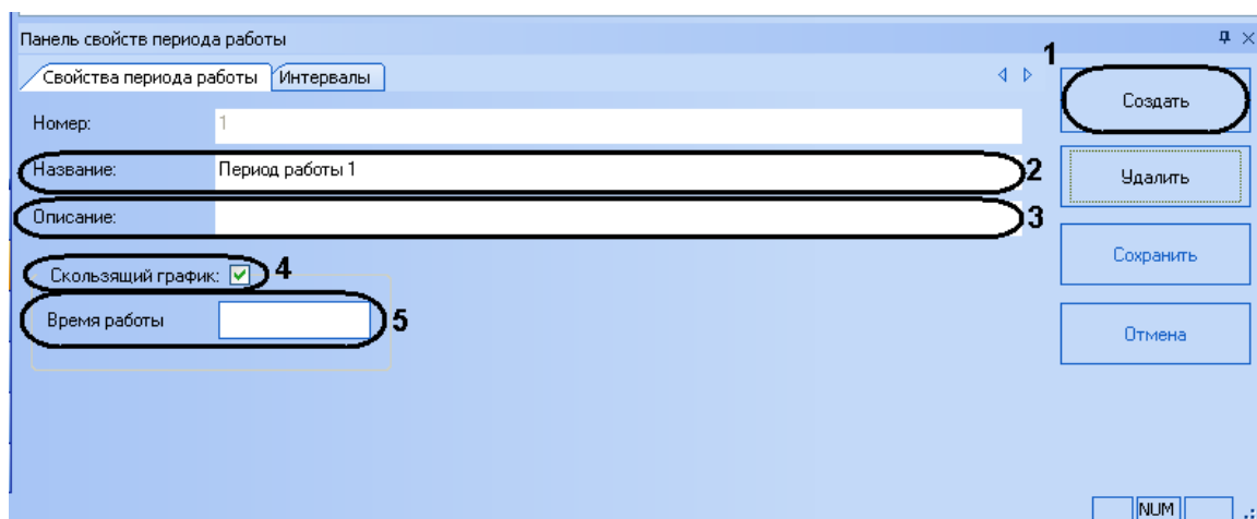
Рис. 7.4—1 Создание периодов работы
