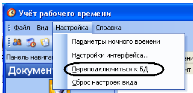
Рис. 6.3—1 Переподключение к базе данных
