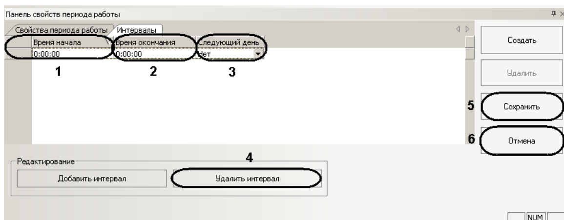
Рис. 7.4—3 Настройка интервала работы
