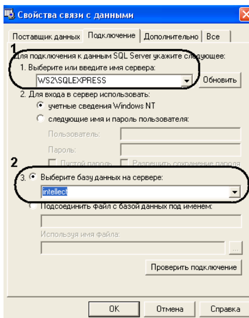
Рис. 4.1—3 Выбор источника данных
