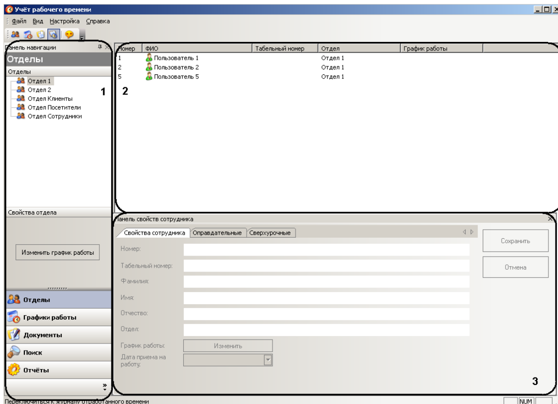
Рис. 5.1—1 Интерфейсное окно модуля Учет рабочего времени
