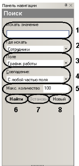
Рис. 7.9—1 Поиск учетных записей
