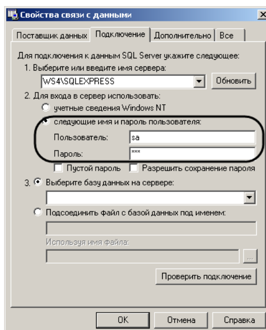
Рис. 4.3—4 Настройка подключения к базе данных с использованием имени пользователя и пароля
