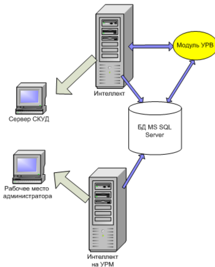
Рис. 4.3—3 Гетерогенная схема из двух и более ядер
