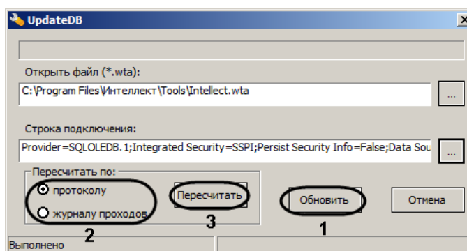
Рис. 9.3—1 Пересчет базы данных
