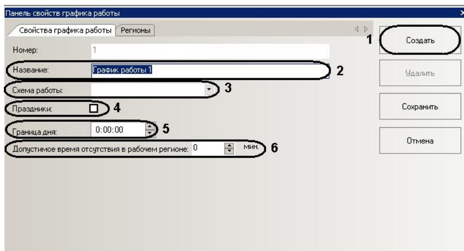
Рис. 7.6—1 Панель свойств графика работы
