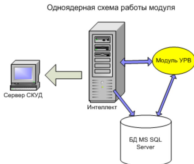
Рис. 4.3—1 Одноядерная схема работы модуля
