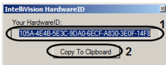
Рис. 6.3—1 Утилита HardwareID.exe
