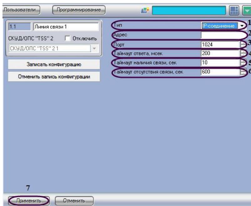
Рис. 3.4—3 Панель настроек подключения СКУД/ОПС TSS2 через Ethernet-соединение
