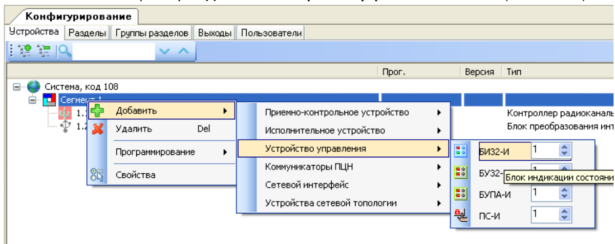
Рис. 3.2—19 Добавление устройств
