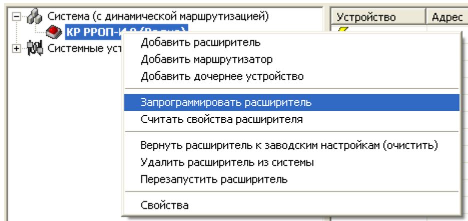
Рис. 3.2—8 Программирование радиорасширителя
