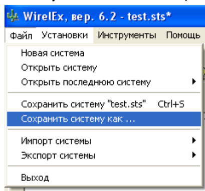
Рис. 3.2—14 Сохранить систему
