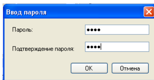
Рис. 3.2—22 Ввод пароля
