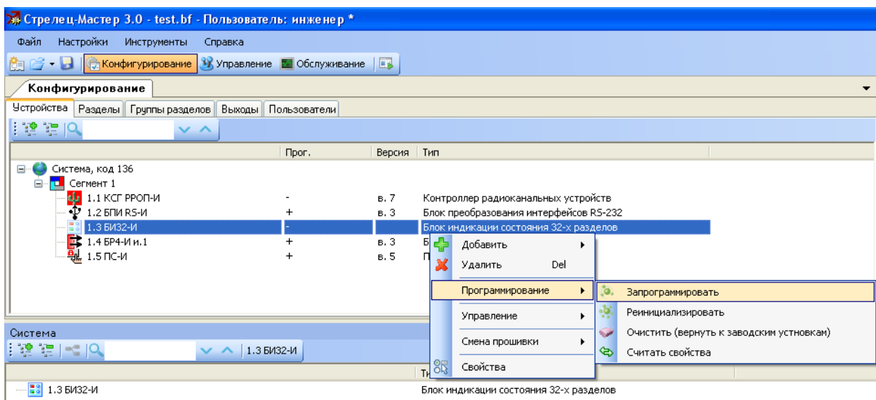
Рис. 3.2—20 Программирование устройств
