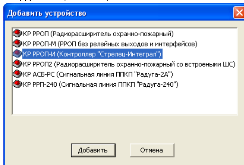
Рис. 3.2—6 Выбор устройства
