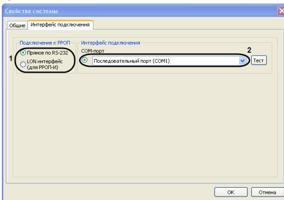
Рис. 3.2—4 Интерфейс подключения
