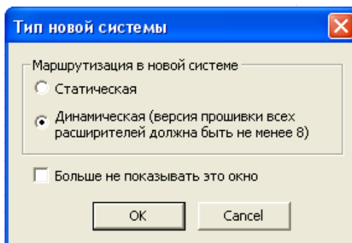
Рис. 3.2—2 Выбор маршрутизации
