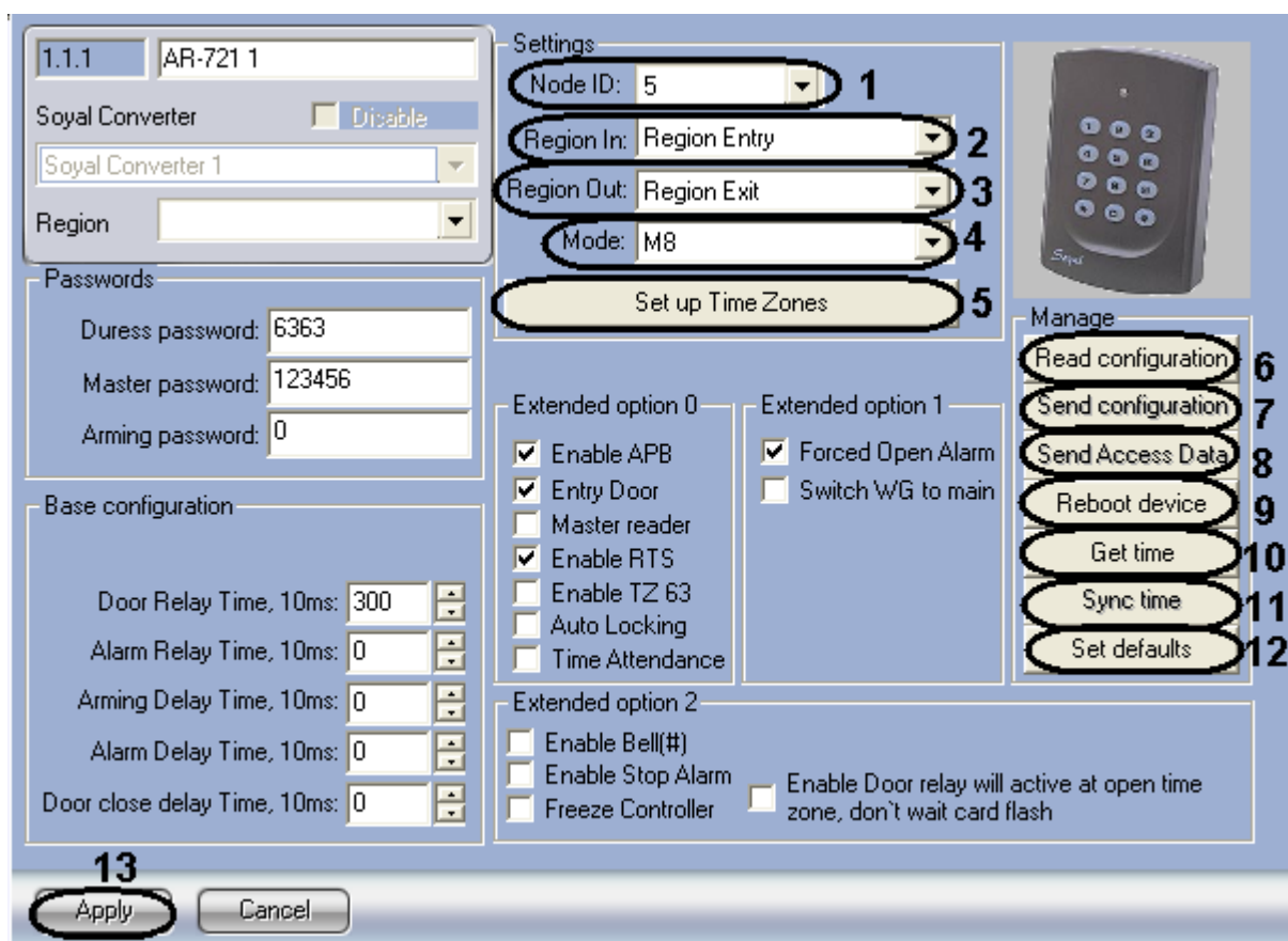
Рис. 2.5—2 Настройка контроллера AR-721
