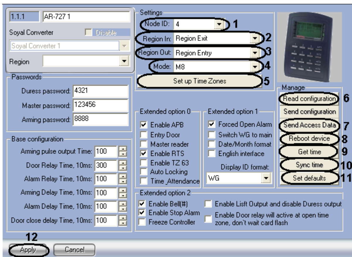
Рис. 2.7—2 Настройка контроллера AR-727
