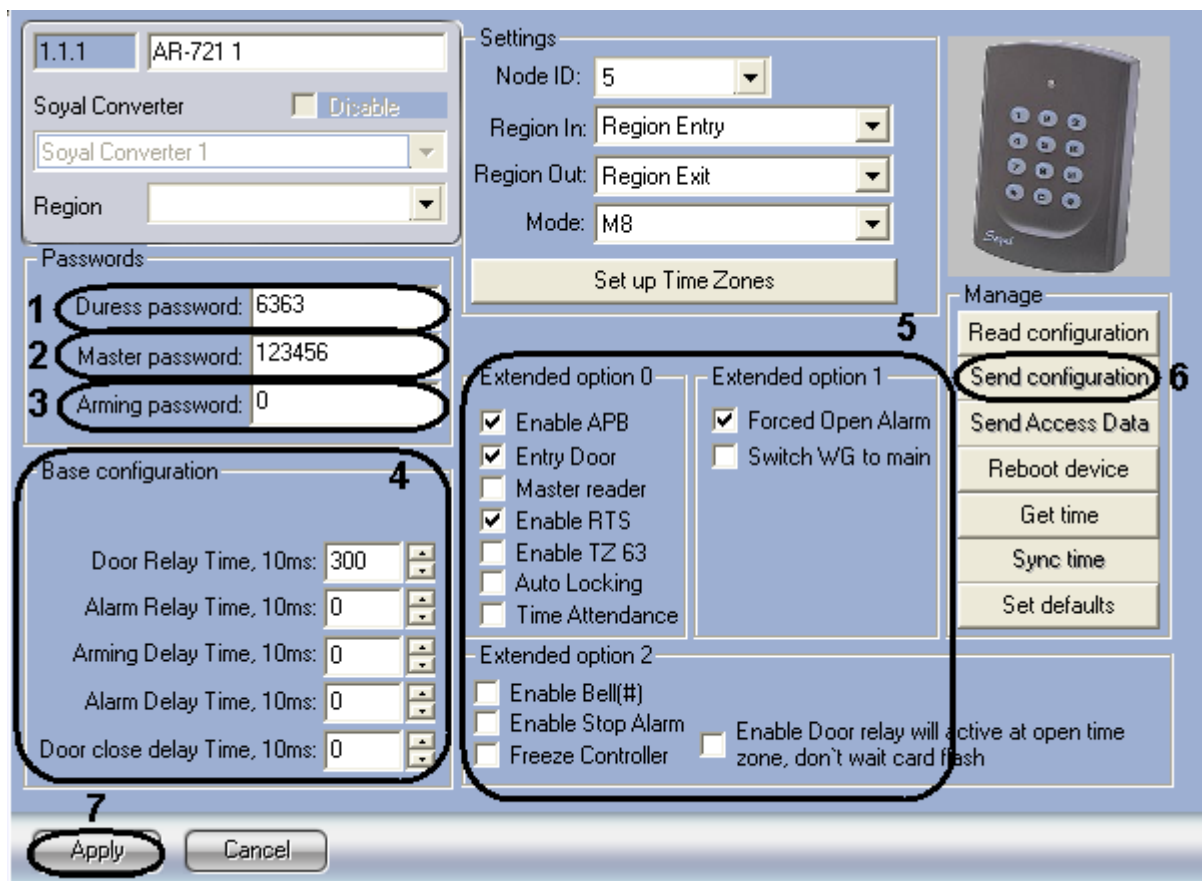
Рис. 2.5—4 Ручная настройка контроллера AR-721
