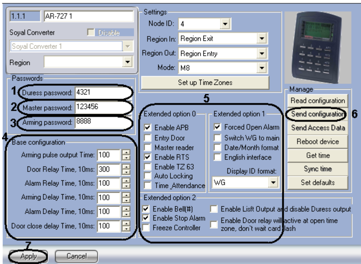
Рис. 2.7—4 Ручная настройка контроллера AR-727
