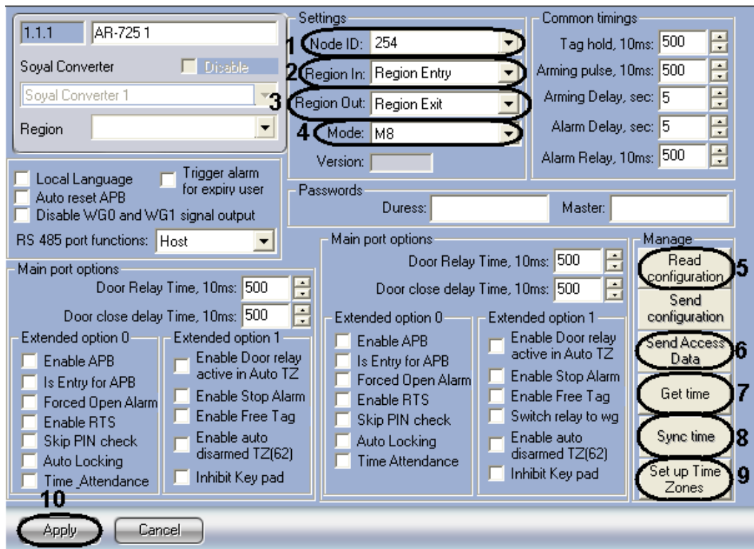
Рис. 2.6—2 Настройка контроллера AR-725
