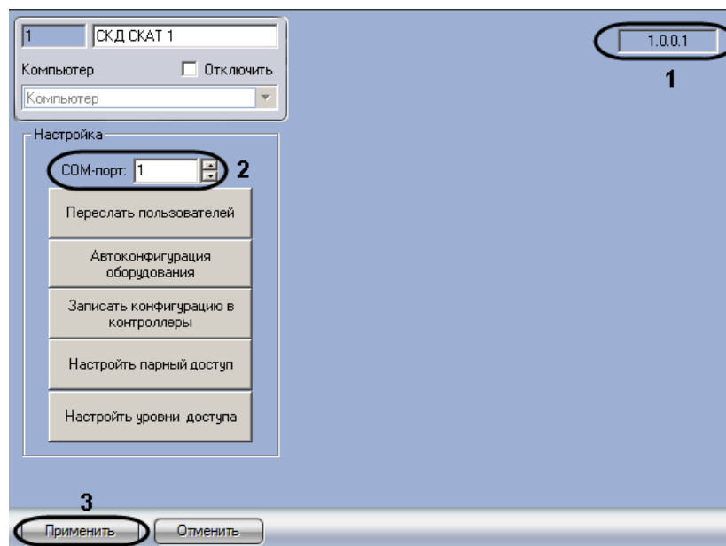
Рис. 3.2—2 Настройка подключения СКУД СКАТ
