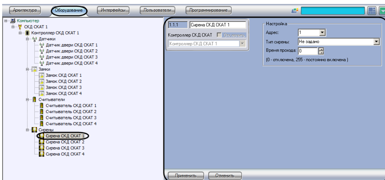
Рис. 3.12—1 Объект Сирена СКД СКАТ
