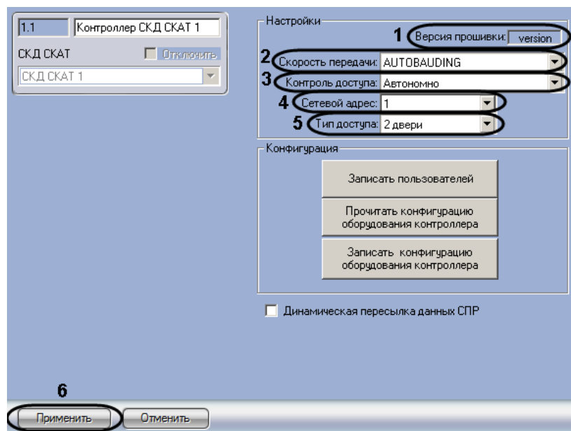
Рис. 3.5—2 Настройка контроллера СКАТ
