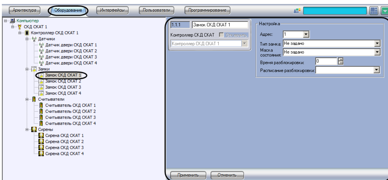
Рис. 3.11—1 Объект Замок СКД СКАТ
