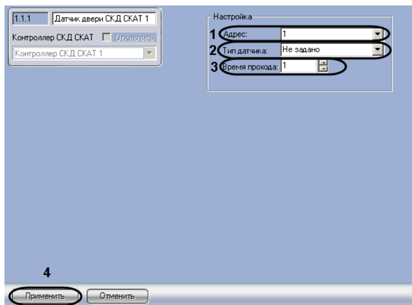
Рис. 3.10—2 Настройка датчика двери СКД СКАТ
