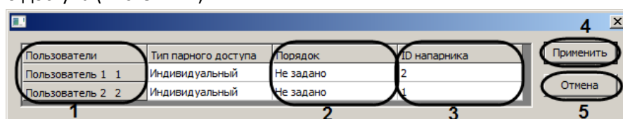
Рис. 3.4—2 Настройка парного доступа
