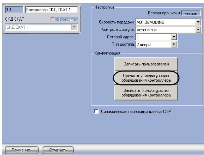
Рис. 3.3—4 Считывание конфигурации контроллера СКАТ
