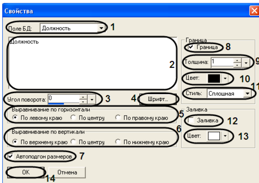
Рис. 3.4—16. Свойства объекта Поле БД
