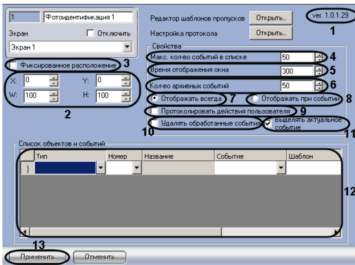
Рис. 3.3—1. Задание параметров модуля Фотоидентификация
