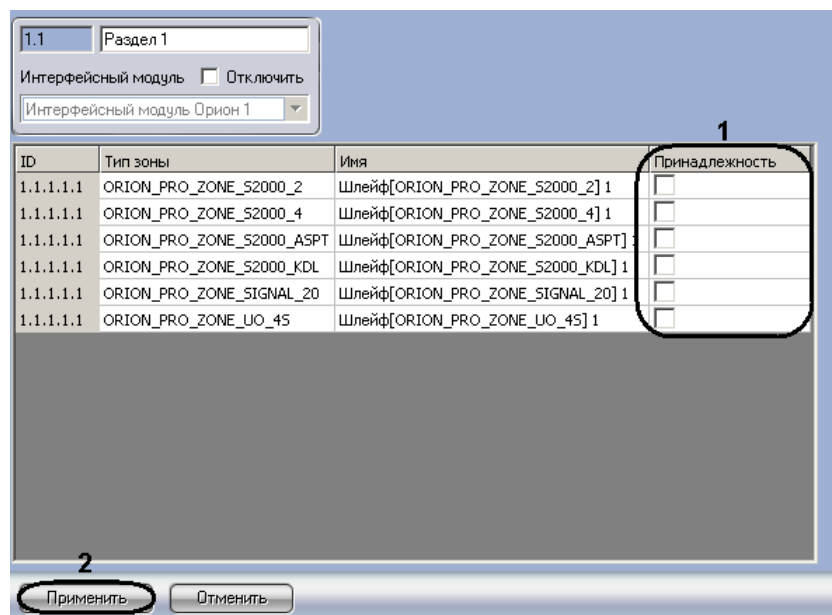
Рис. 3.3—13 Панель настроек объекта Раздел
