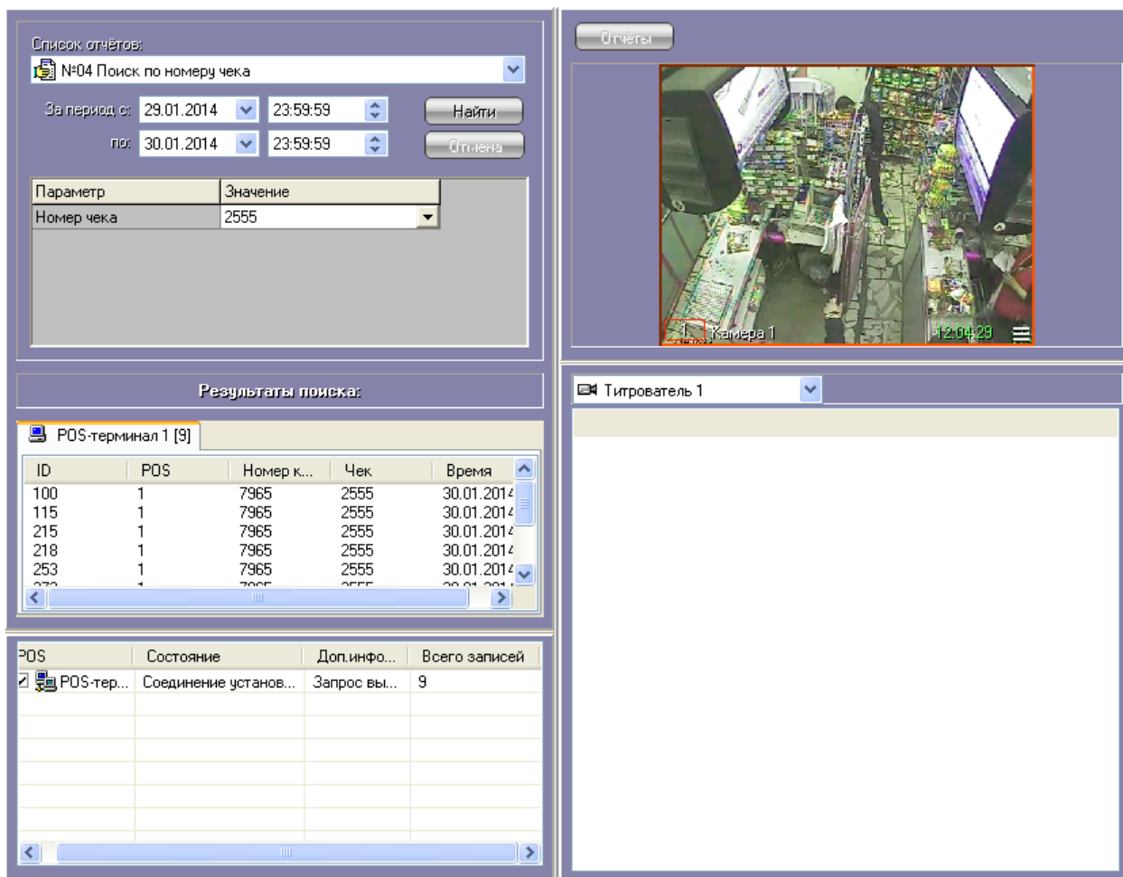
Рис. 4.4-16. Изменение размеров элементов (исходное состояние)
