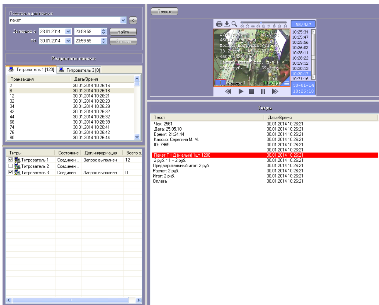
Рис. 5.2-1. Интерфейс объекта «Поиск по титрам»
