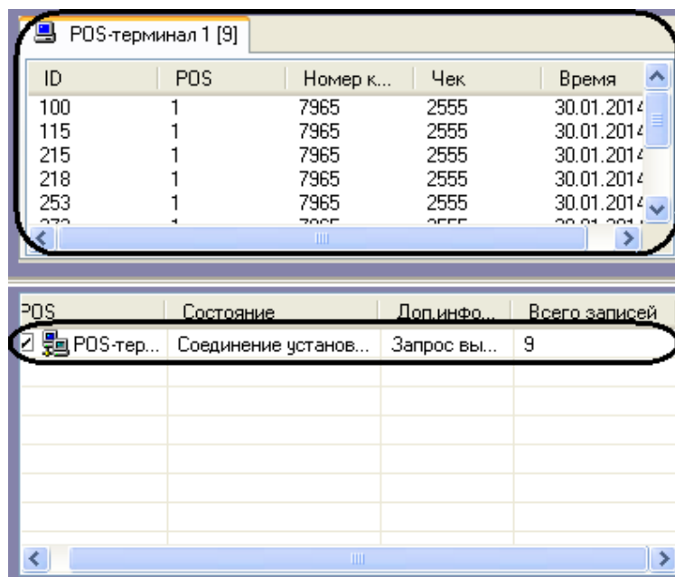
Рис. 4.4-8. Окончание поиска
