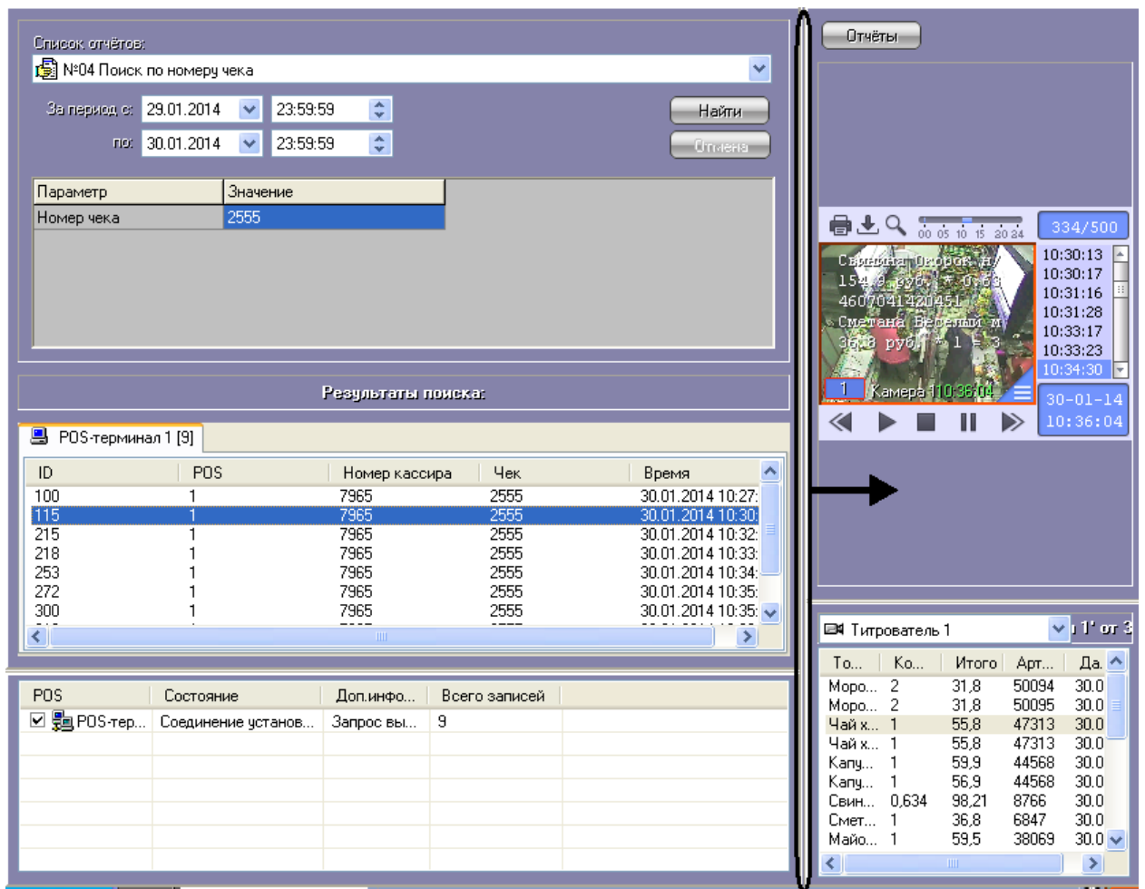
Рис. 4.4-18. Изменение размеров элементов (одновременный сдвиг по горизонтали)
