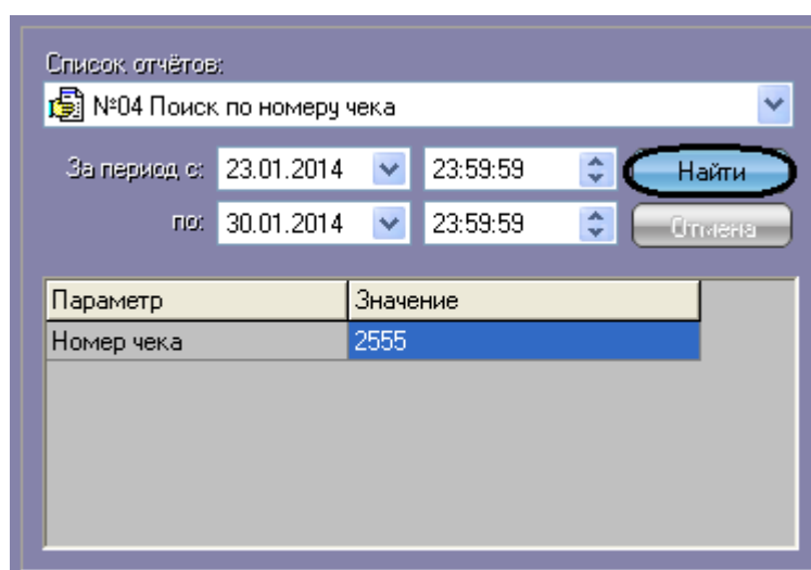
Рис. 4.4-5. Запуск поиска
