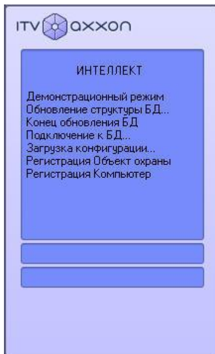
Рис. 4.1-1. Запуск Программы
