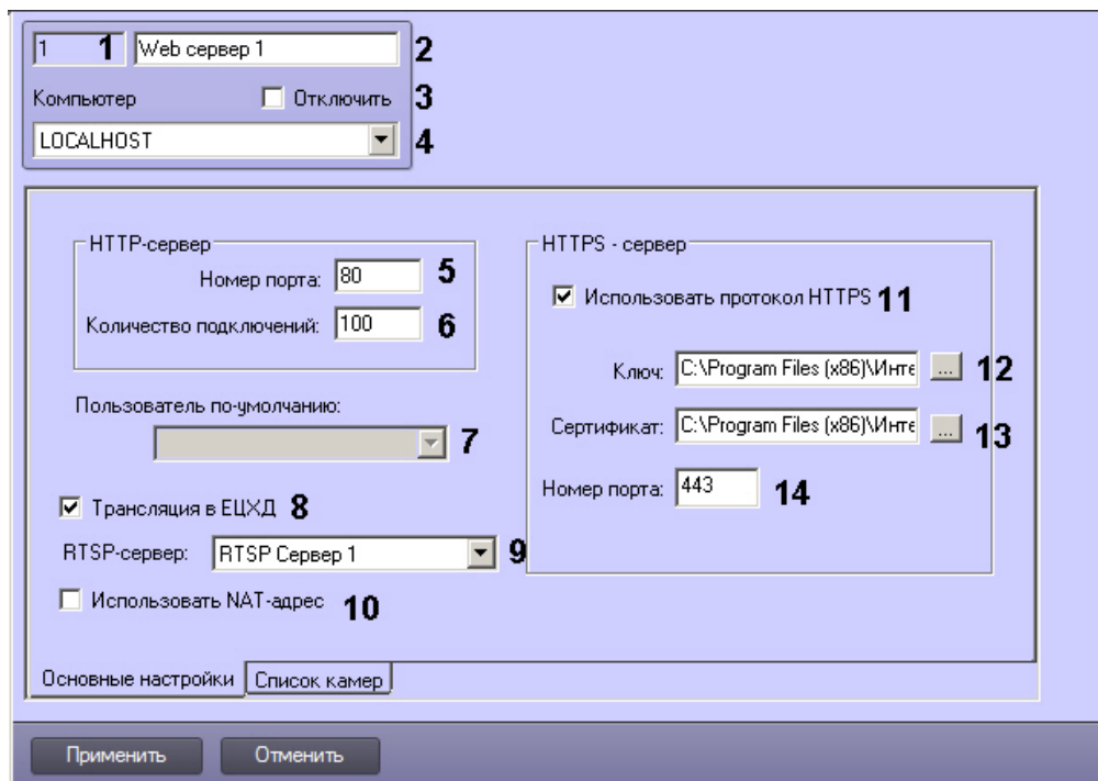
Вкладка Основные настройки
