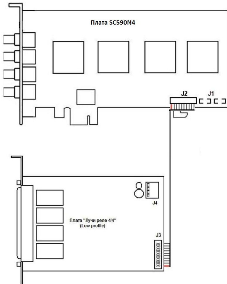
Схема подключения платы лучи-реле 4/4 (low profile) к плате SC590N4
