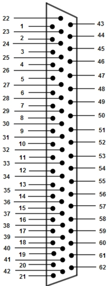
Разводка внешнего разъема плат SL USBIO 16x8 и USBIO 2 4x4
