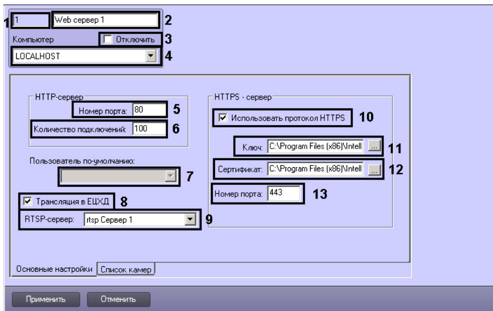
Вкладка Основные настройки
