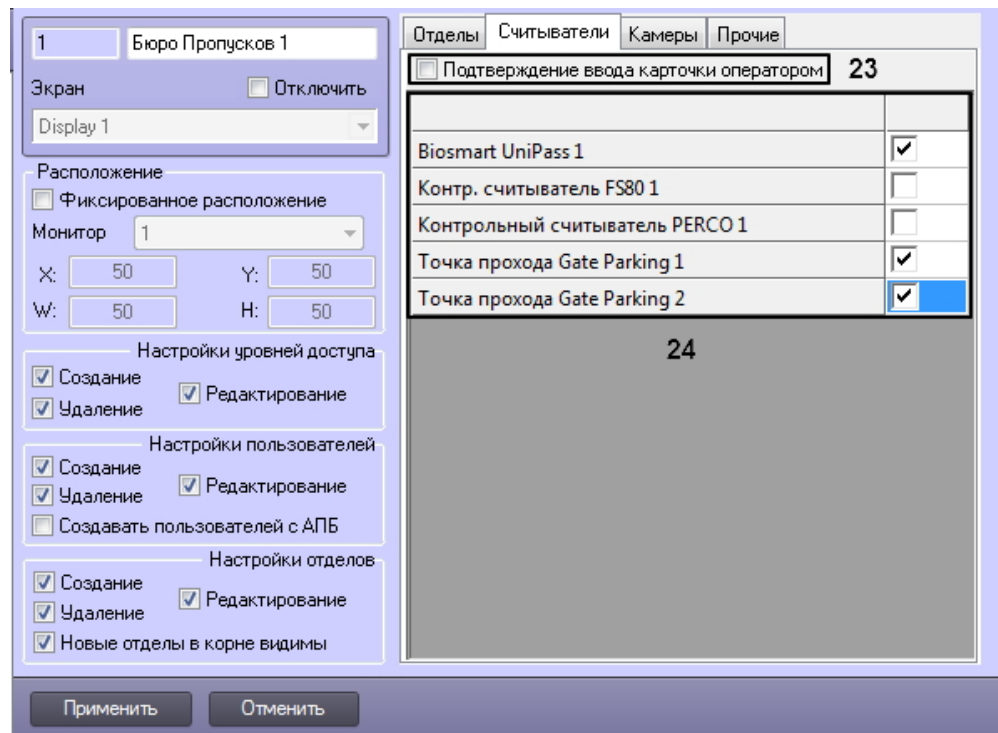
Вкладка Считыватели
