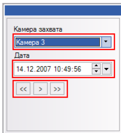
Рис. 4.2-24 Панель навигации по фотоархиву
