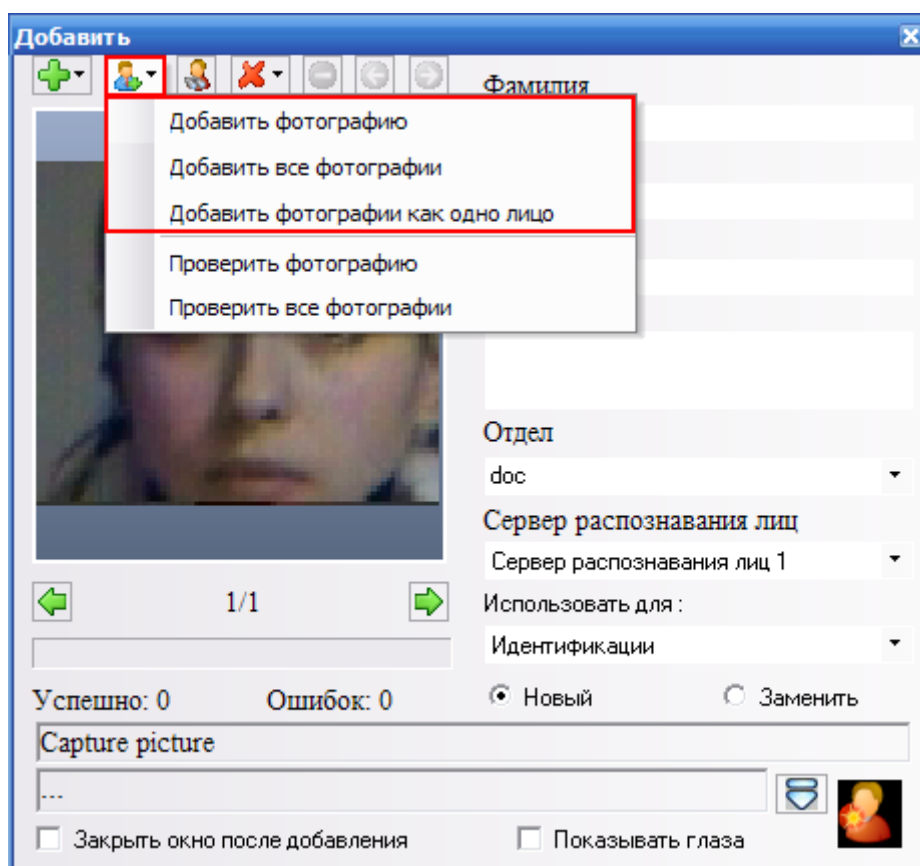
Рис. 4.2-11 Добавление фотографий (меню)
