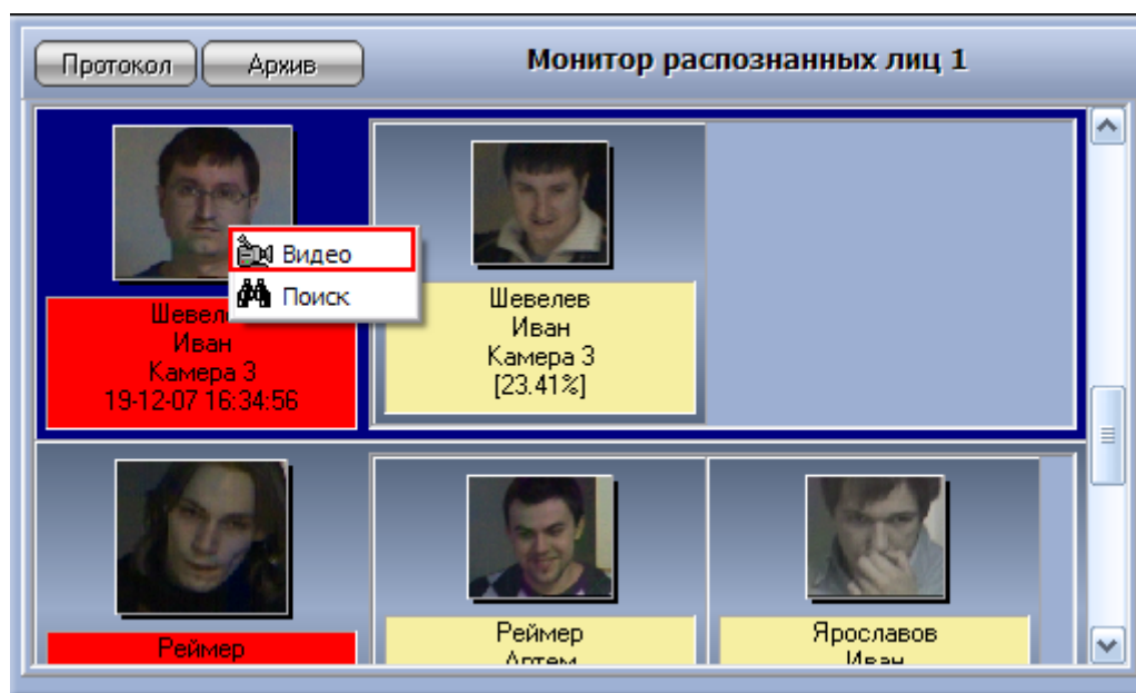
Рис. 4.3-7 Просмотр видеофрагмента, соответствующего распознанному лицу (вкладка «Протокол»)
