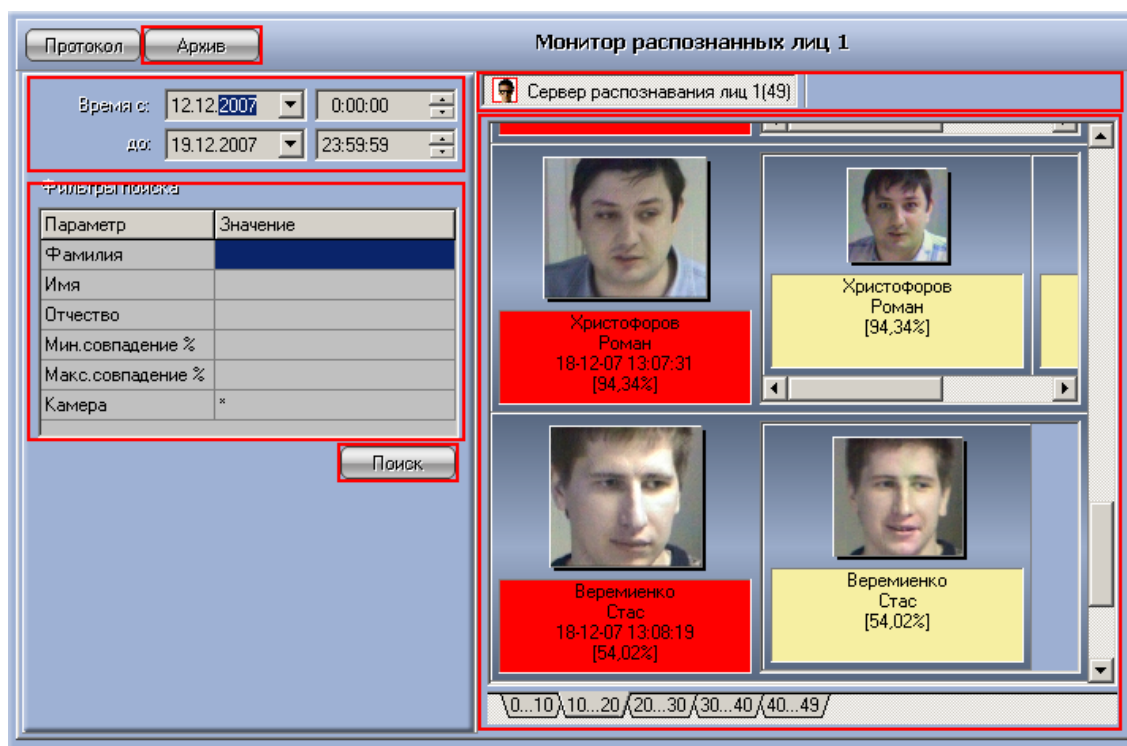
Рис. 4.3-6 Поиск распознанных лиц (вкладка «Архив»)
