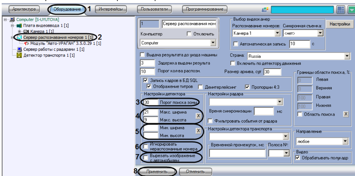
Рис. 7.2—26. Настройка детектора
