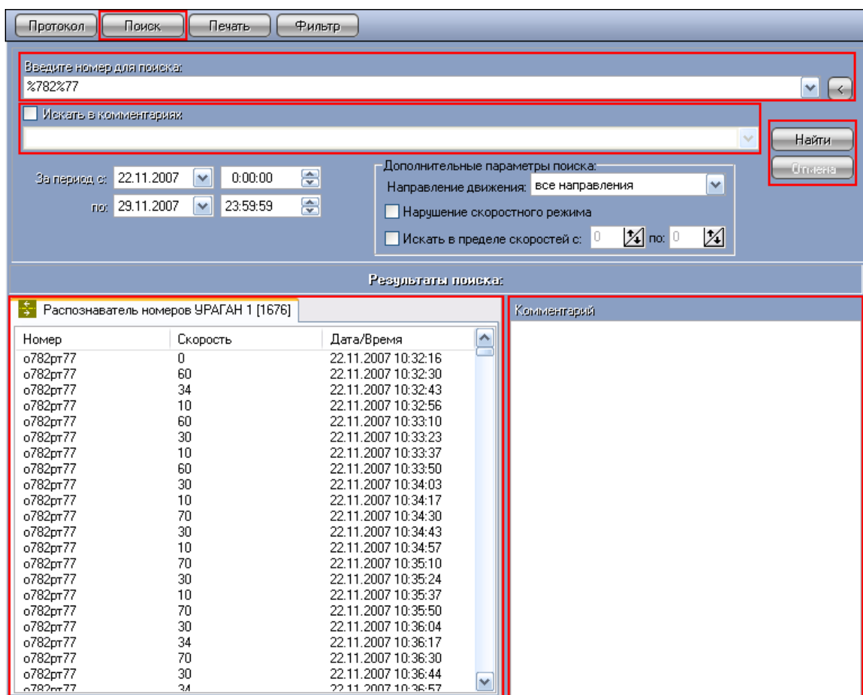
Рисунок 4.2.6-1 Доступ к полной информации о распознанном номере
