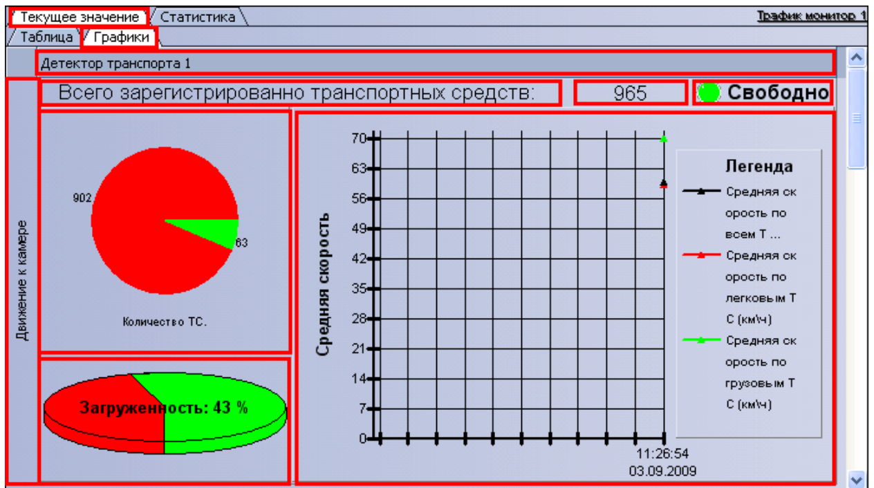
Рисунок 5.2.2-2 Внешний вид интерфейса панели «Графики» вкладки «Текущее значение» (отображение по направлениям)
