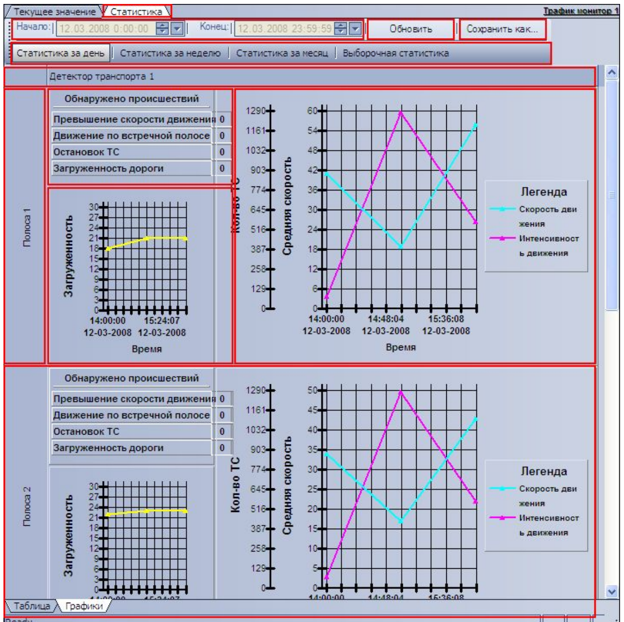
Рисунок 5.2.4-1 Внешний вид интерфейса панели «Графики» вкладки «Статистика»
