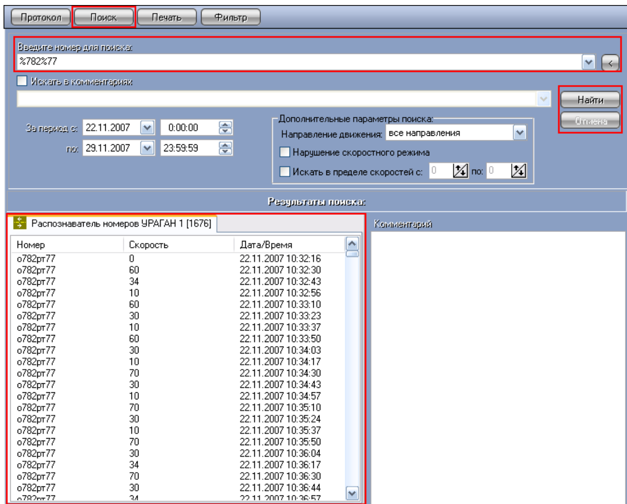
Рисунок 4.2.2-1 Просмотр кадра видеозаписи, соответствующего моменту определения номера
