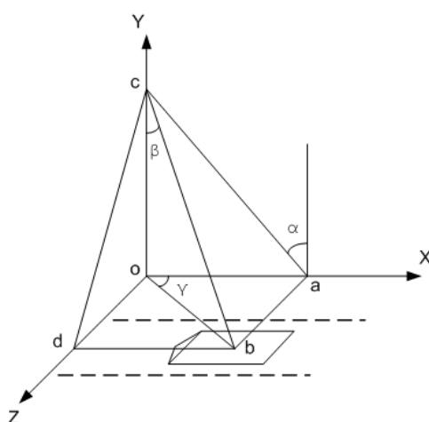
Рис. 6.2—6. Геометрия зоны детектирования
