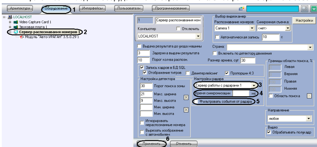
Рис. 7.2—20. Настройка совместной работы Сервера распознавания номеров и программного модуля «Радар»
