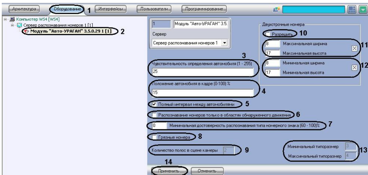
Рис. 7.2—3. Настройка программного модуля «Авто-УРАГАН 3.5.0.29»
