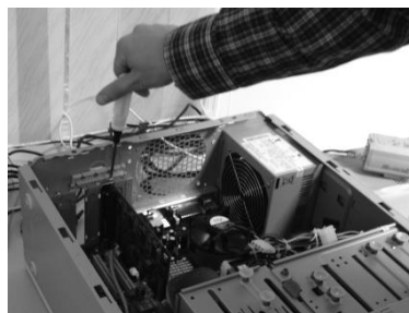
Рис. 3.1—2. Пример установки платы видеоввода в PCI слот
