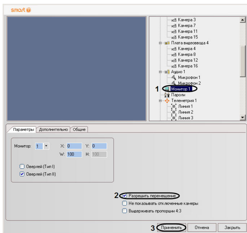
Рис. 5.2—6. Ввод запрета на перемещение монитора видеонаблюдения
