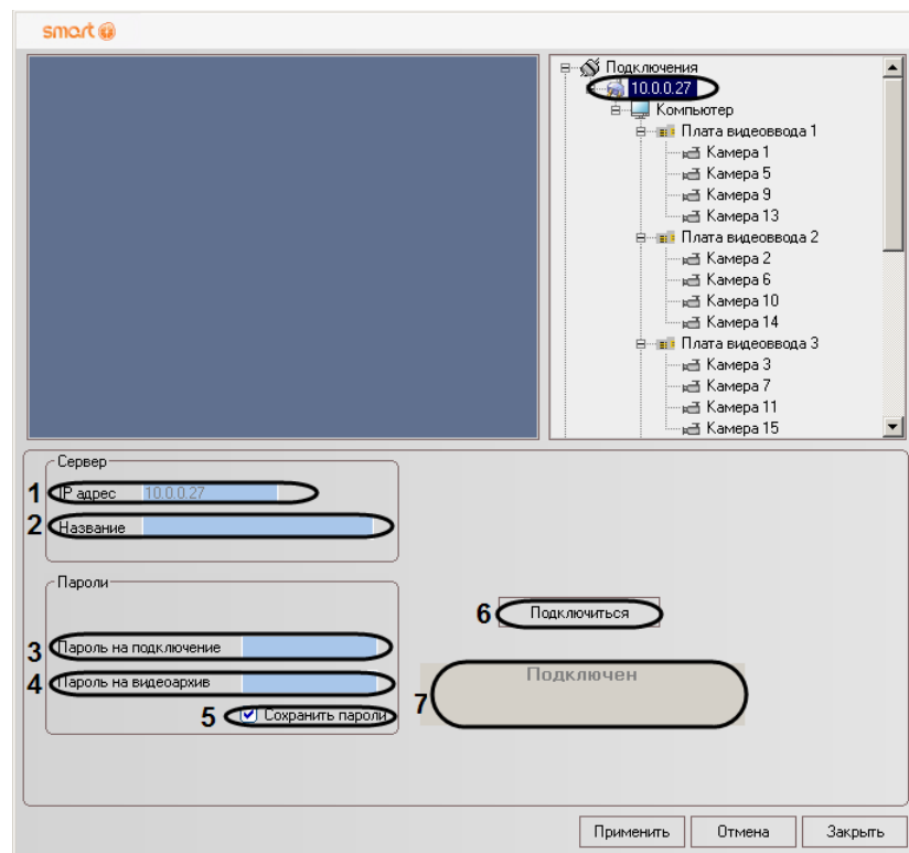
Рис. 10.2—2. Панель настройки объекта «IP-адрес сервера»
