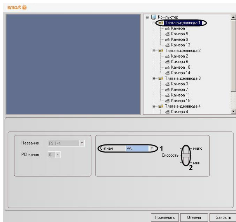
Рис. 9.4—4. Панель настройки объекта «Плата видеоввода»
