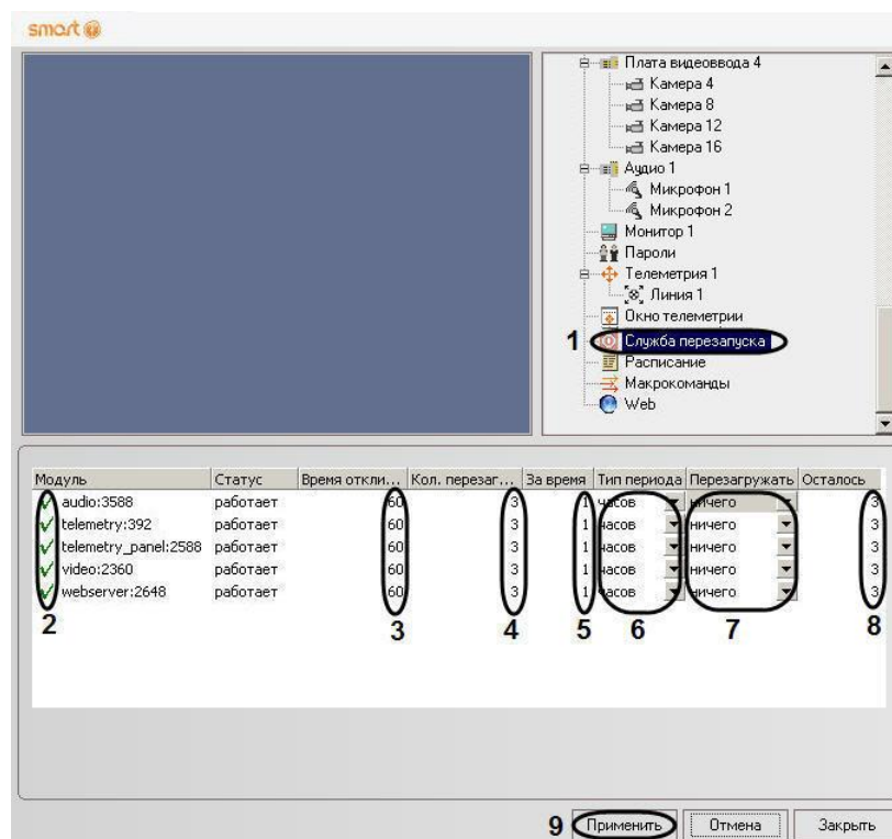
Рис. 5.2—44. Настройка Службы перезагрузки системы
