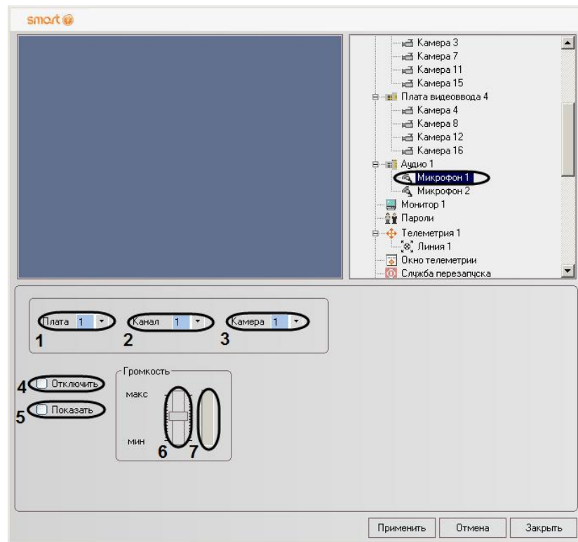
Рис. 9.4—10. Панель настройки объекта «Микрофон»
