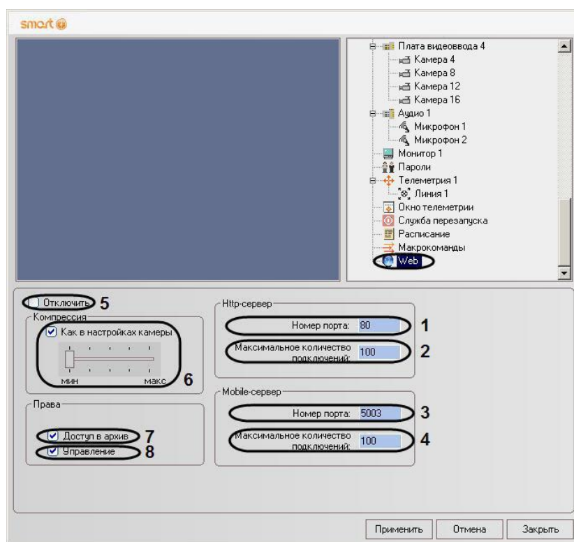
Рис. 5.4—1. Панель настройки объекта «Web»
