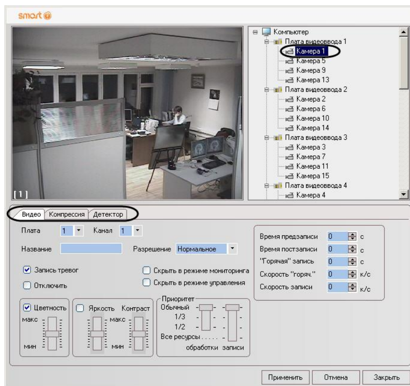
Рис. 9.4—5. Вкладки панели настроек объекта «Камера»
